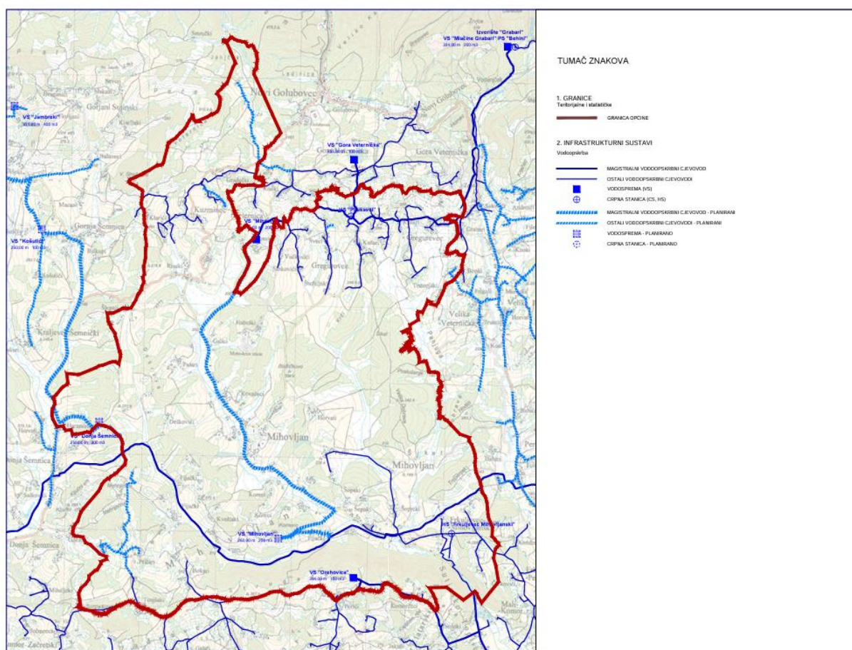
Slika 28. Razgranatost vodoopskrbne mreže na području Općine Mihovljan Izvor: Prostorni plan uređenja Općine Mihovljan
